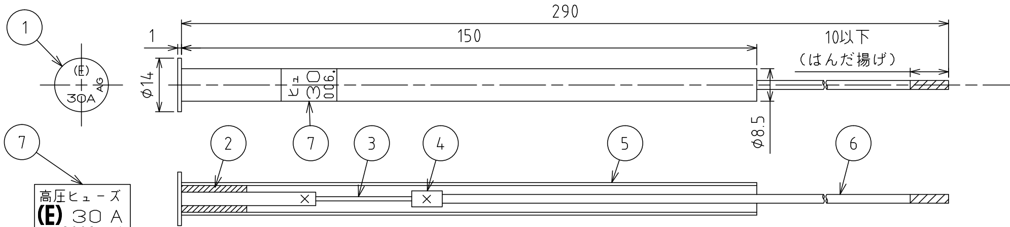
半断面図
