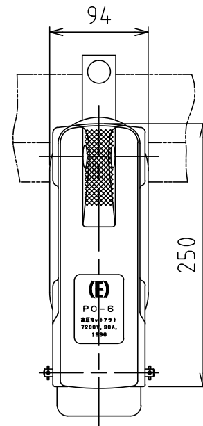
A-A 視図
