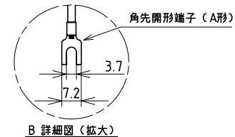
B 詳細図 (拡大)
